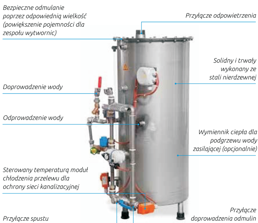
Ilustracja: Zbiornik odmuliania, konfiguracja przykładowa
